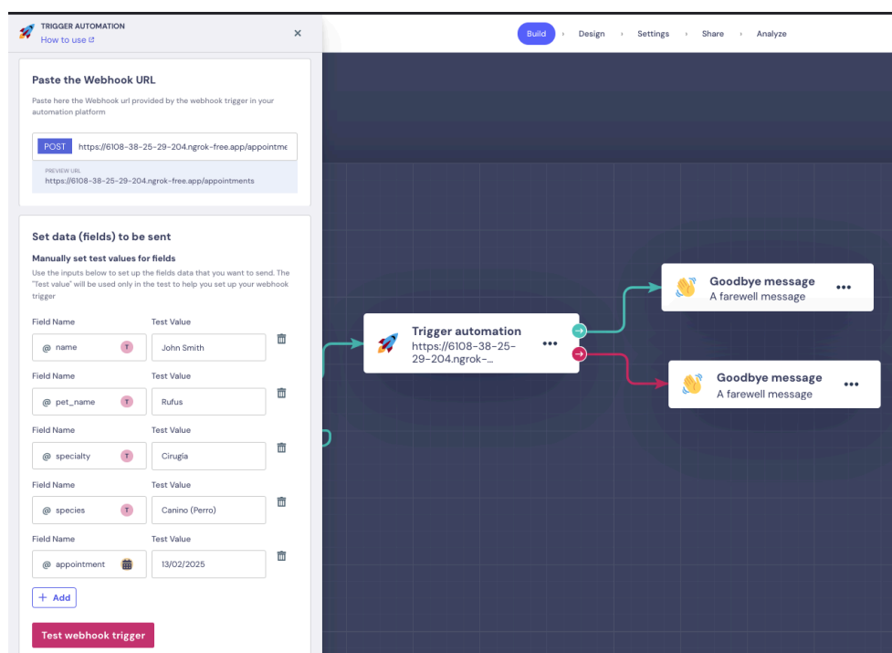
Figura 6. Nodo de automatización para conectarse al servicio de citas.
