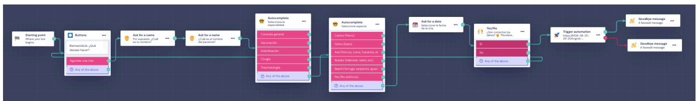
Figura 5. Sistema de construcción basado en nodos de Landbot.
